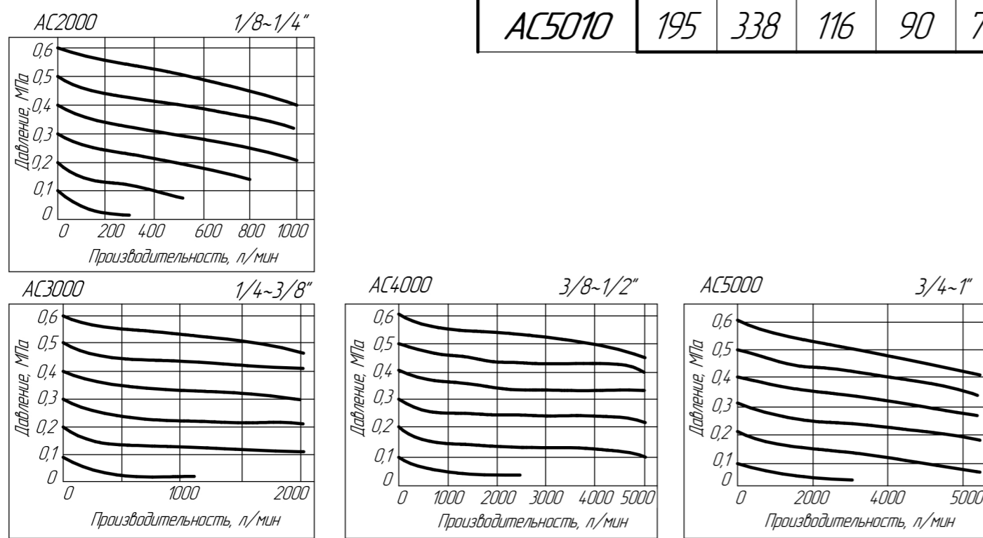
Кривые расхода воздуха
